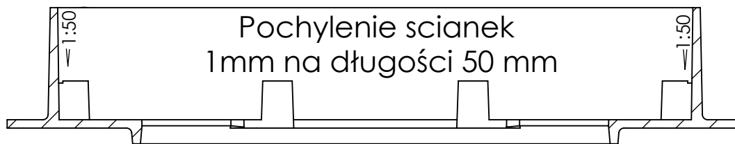
PRZEKRÓJ A-A SKALA 1 : 5
